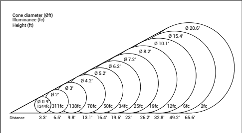
ODESSA 2-G (Medium)
