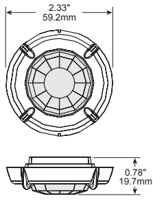
FSP-L2 dimensions
